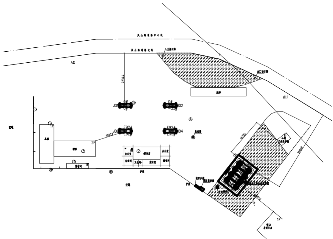
图 2-1 加油站总平面布置图
