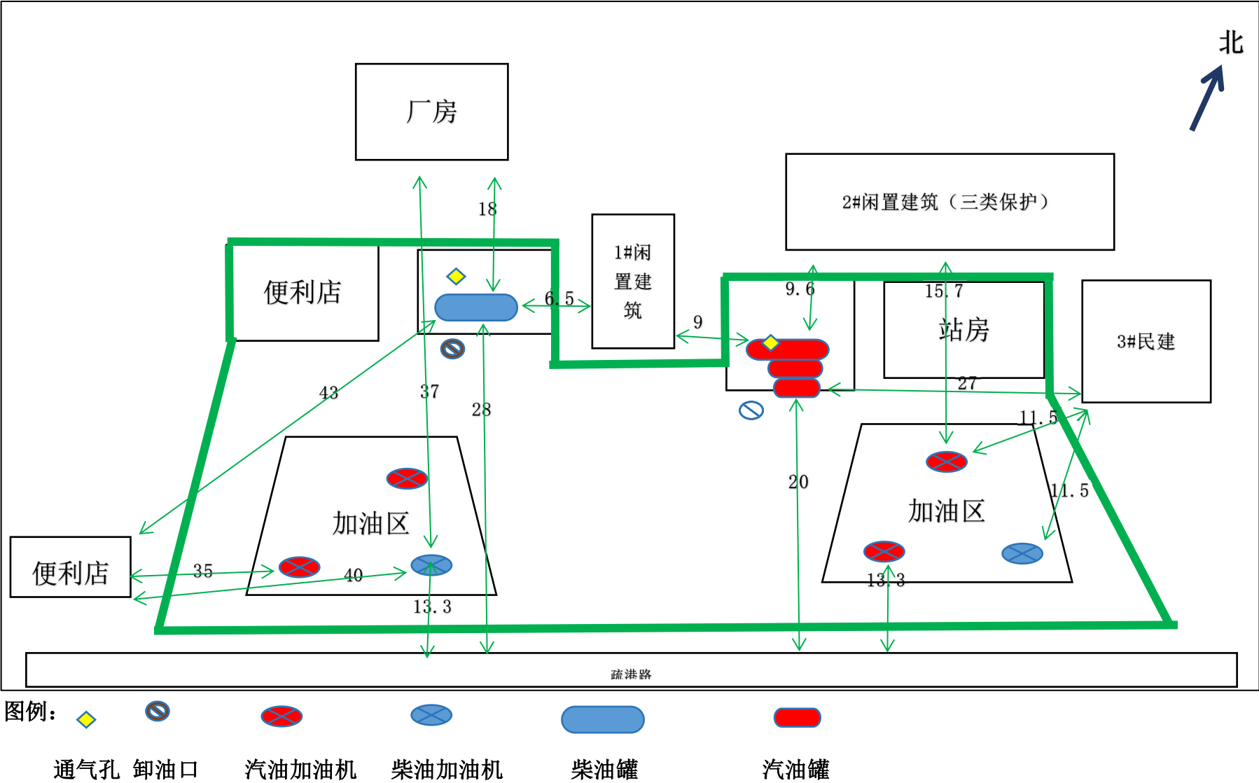
图2-2 加油站平面示意图
